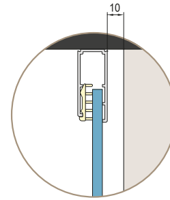
Fig. 2 Paroi fixe
