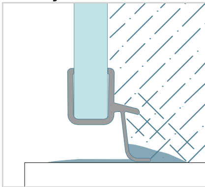
Parois de douche sans cadre et sans barre de seuil
