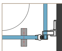
Détail A vue de dessus :
