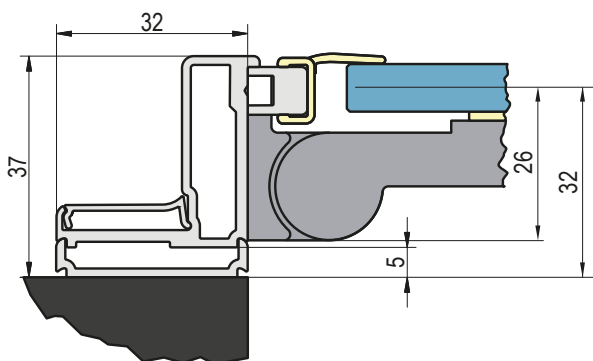
Profilé de fixation murale utilisé pour porte ou paroi fixe PUR
