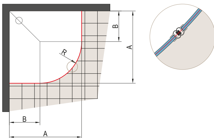
A | Dimension mesurée du mur, carrelage posé, à la position réelle de la paroi.
