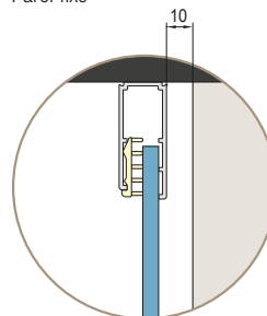
Fig. 2 Paroi fixe
