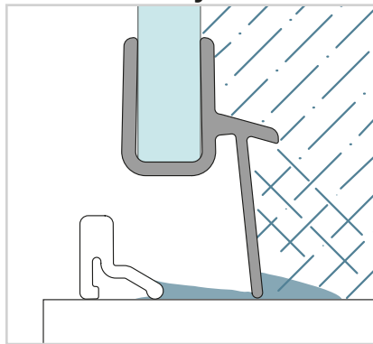
Parois de douche avec profilés et profilé de seuil moyen
