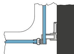
Détail A vue de dessus :
