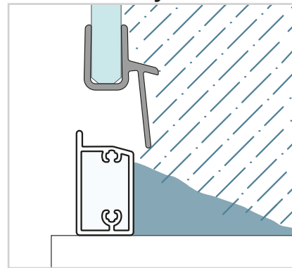
Parois de douche avec profilé de cadre
