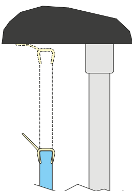
Nischentür
