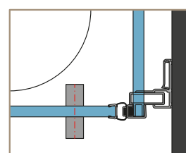
Detail A - Draufsicht
