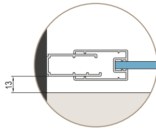
Bild 1 Türen, Eckeinstieg, Runddusche
