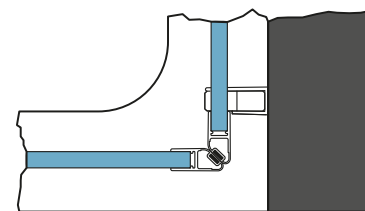
Detail A Draufsicht:
