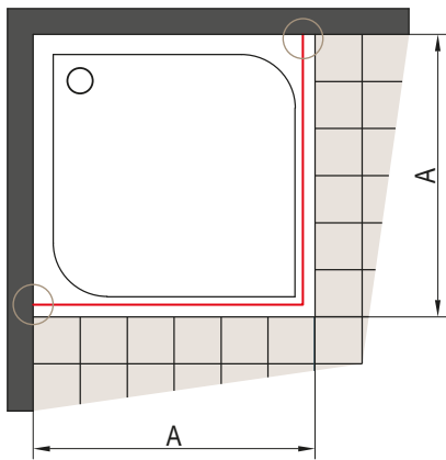
Bild 1 Türen, Eckeinstieg, Runddusche
