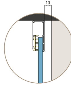
Bild 2 Seitenwand
