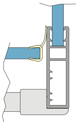
Tür + Seitenwand
