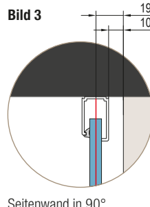
Seitenwand in 90°
