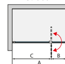
D22WI3 mit horizontaler Stabilisationsstrebe
