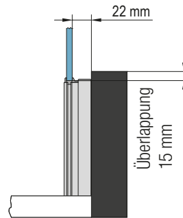
Detail A Frontansicht:
