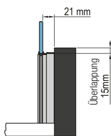
Detail A - Frontansicht
